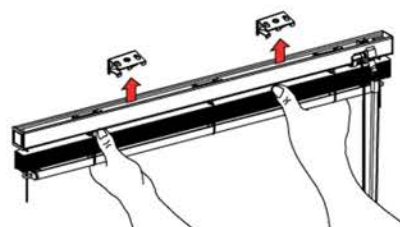
plaatsing van de montagebeugels op de bovenbak
