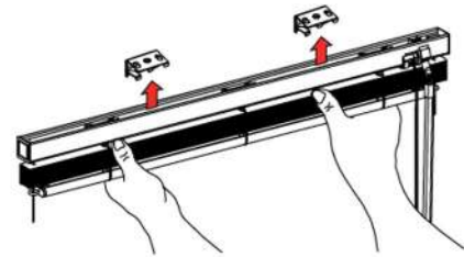
plaatsing van de montagebeugels op de bovenbak
