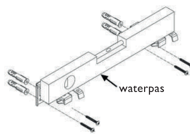
op de dag (bijv. wandmontage)
