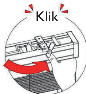
vastklemmen beugels met borging
