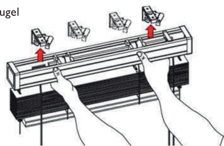
plaatsing van de bovenbak op de montagebeugels
